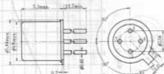
(JEDEC TO-72)
