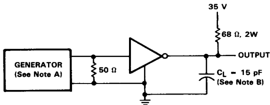
TEST CIRCUITS
